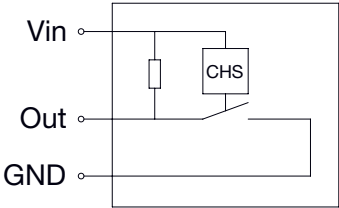
Anschlusschema CHS1 (Ohne Beleuchtung)
