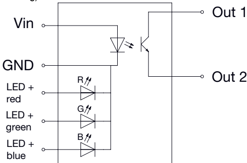
Anschlusschema CHS2 und CHS3 (Mit Beleuchtung)
