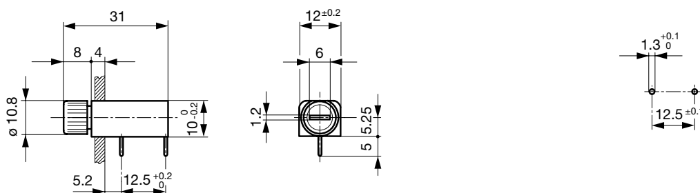
Bohrplan
