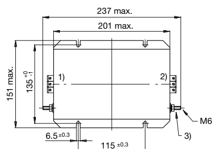
Gehäuse 32-C
