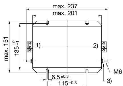
Gehäuse 34-C
