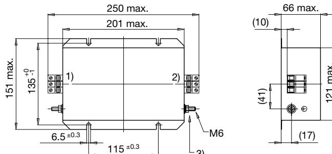
Gehäuse 37-3
