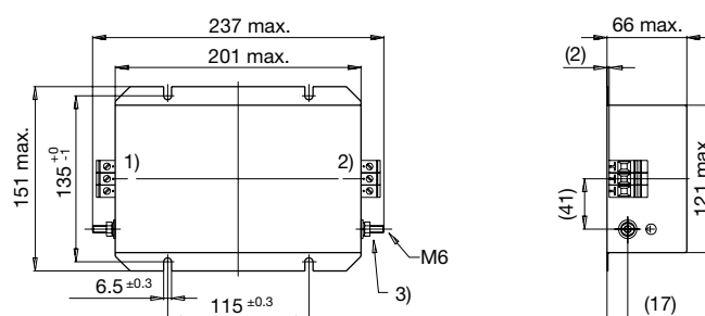
Gehäuse 34-3
