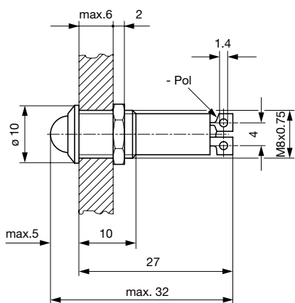
LFM mit vorstehender LED und Vorwiderstand und Aussenreflektor
