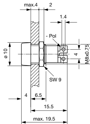
LFM ohne Vorwiderstand mit Innenreflektor
