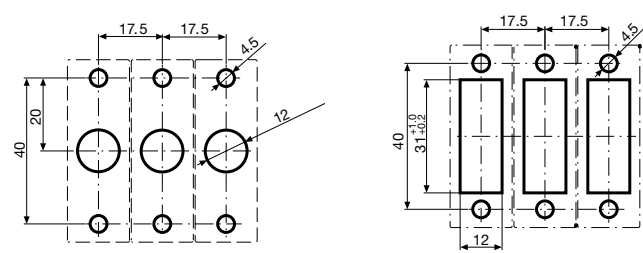
Montage von hinten Montage von vorne
