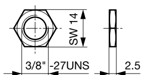
Sechskantmutter TZZ12 / TZZ51
